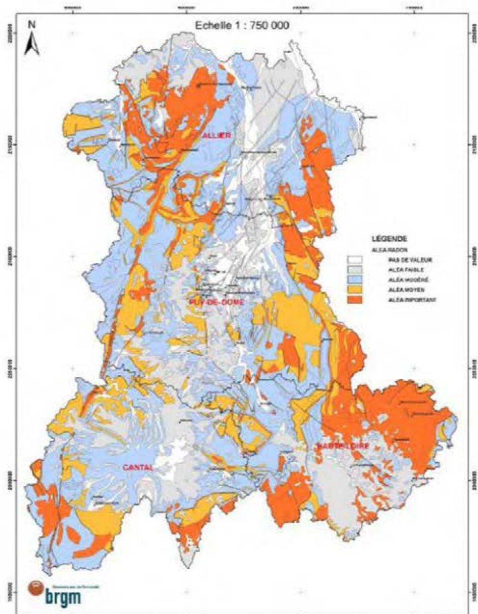
Illustration 17 - Aléa radon estimé à partir de l'ensemble des indications de potentiel uranium : teneurs moyennes en uranium des formations géologiques, indices d'uranium, failles et permis d'exploration minière
